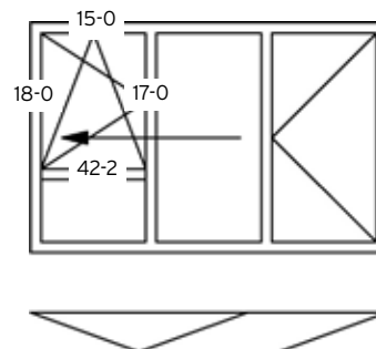
Faltwand mit Dreh-/Kippflügel im Faltflügel oberhalb Querkämpfer. Folding façade with tilt and turn window above transom integrated in folding door panel.
